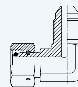
DIN 2353 Swivel Adjustable 90° Elbow JIC Male
