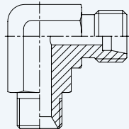
DIN 2353 90° Elbow BSPP Male
